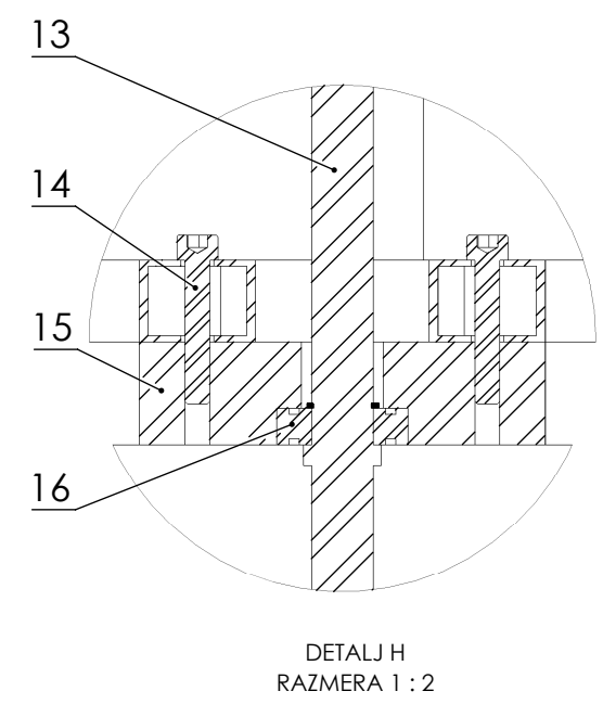
DETALJ H RAZMERA 1 : 2
