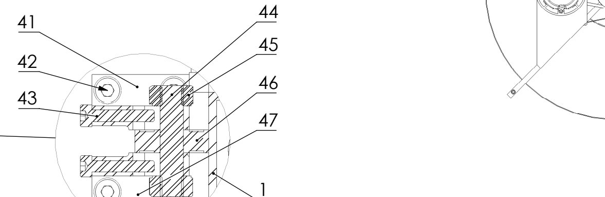
DETALJ K RAZMERA 1 : 1
